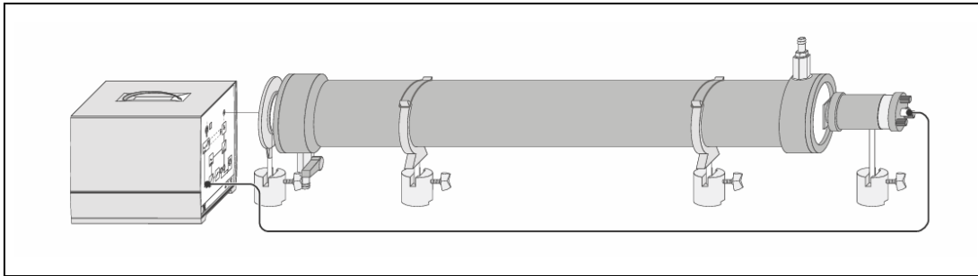
Fig. 5. Determinación de la velocidad de la luz en agua.
